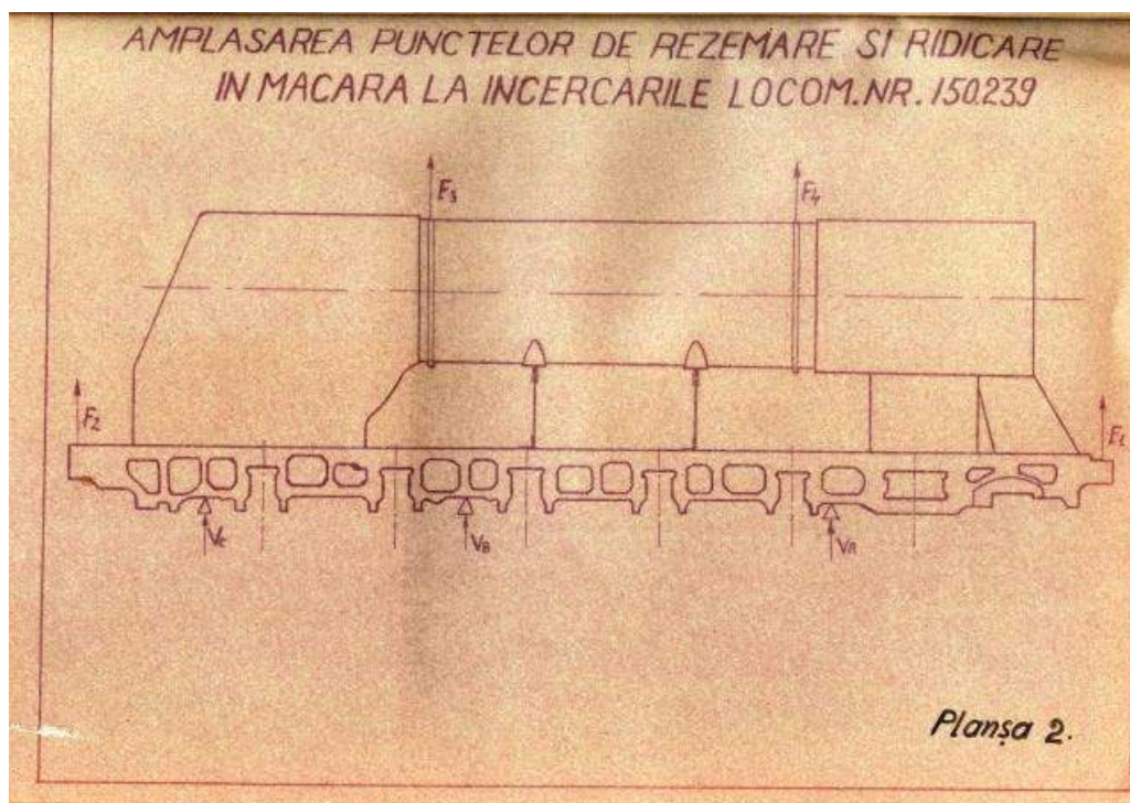
Fig. 5 Amplasarea punctelor de rezemare și ridicare
