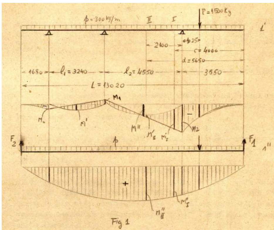
Fig. 6 Diagramele de eforturi pentru Lonjeronul considerat ca grindă continuă pe 3 reazeme
